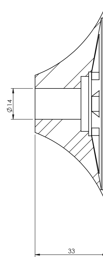
SEZIONE C-C
